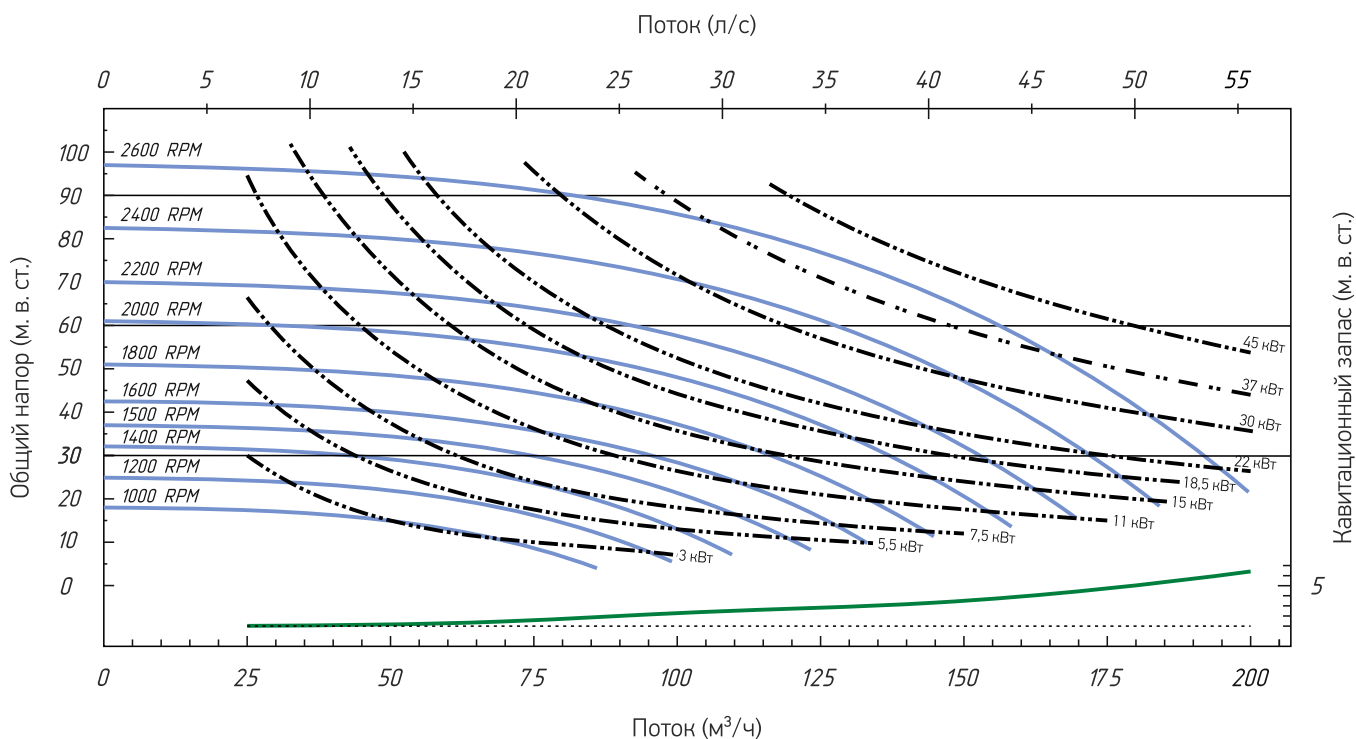
Рабочая характеристика насоса при плотности рабочей среды 1000 кг/м³
